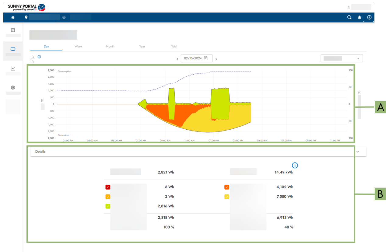
Abbildung 13: Übersicht der Energiebilanz einer Sunny Home Manager Anlage
