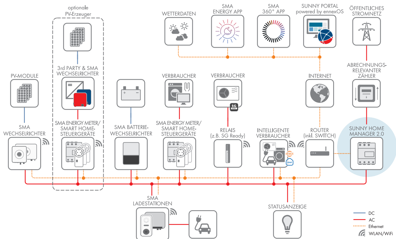
Abbildung 4: Betrieb der PV-Anlage mit SMA Wechselrichtern
