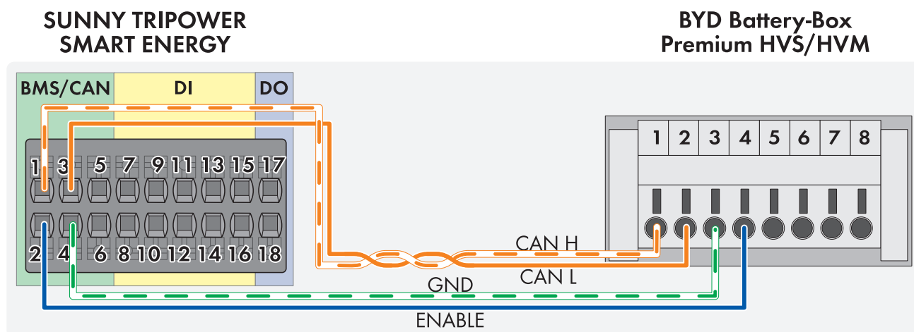
Abbildung 2: Verkabelungsprinzip nach TIA-568B: Sunny Tripower Smart Energy mit BYD Battery-Box Premium HVM/HVS bei Verwendung von Verlegeleitung. Die einzelnen Leitungsenden müssen mit einer 12mm langen Adernendhülse versehen sein.
