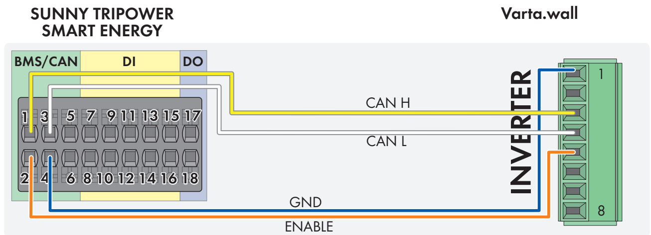
Abbildung 7: Sunny Tripower Smart Energy mit Varta.wall. Sofern keine Verlegeleitung verwendet wird, müssen die einzelnen Leitungsenden mit 12 mm langen Aderendhülsen versehen sein.
