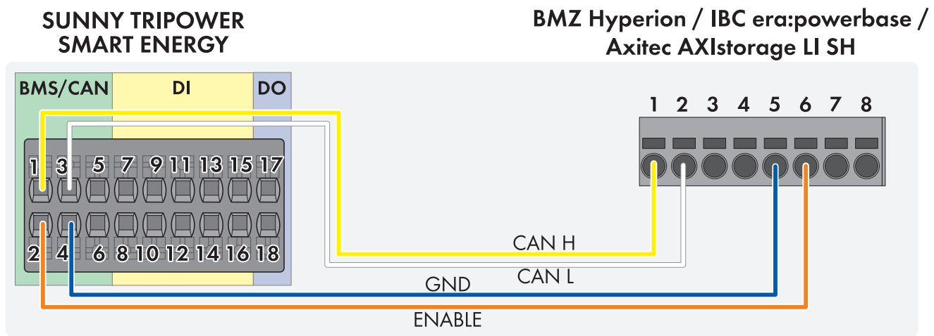
Abbildung 6: Sunny Tripower Smart Energy mit BMZ Hyperion, AXITEC AXIstorage, IBC era:powerbase bei Verwendung des vom Batteriehersteller mitgelieferten Kommunikationskabels. Sofern keine Verlegeleitung verwendet wird, müssen die einzelnen Leitungsenden mit 12 mm langen Aderendhülsen versehen sein.
