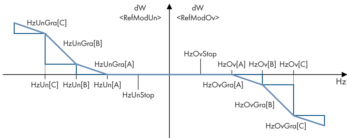
Abbildung 21: Beispiel einer P(f)-Kennlinie
