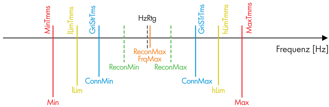
Abbildung 20: Frequenzüberwachung (HzRtg: Nennfrequenz des öffentlichen Stromnetzes)
