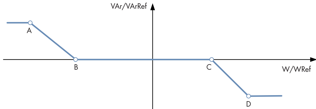
Abbildung 10: Beispiel einer Q(P)-Kennlinie für Erzeuger und Verbraucher mit 4 Stützpunkten
