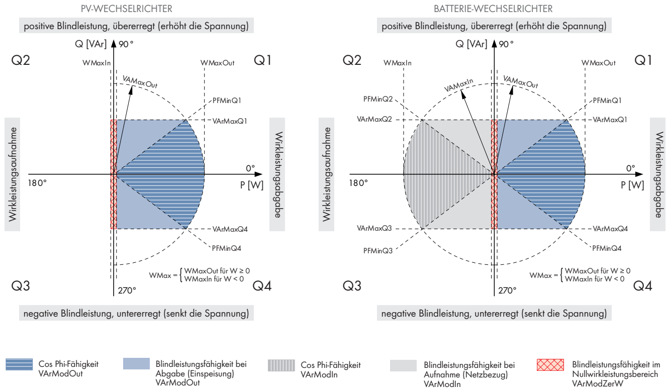
Abbildung 3: Nenngrößen und Blindleistungsbereiche im P/Q-Diagramm im Erzeugerzählpeilsystem für PV- und Batterie-Wechselrichter
