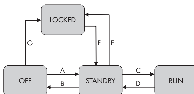
Abbildung 4: Übersicht der Betriebszustände mit Zustandsübergängen
