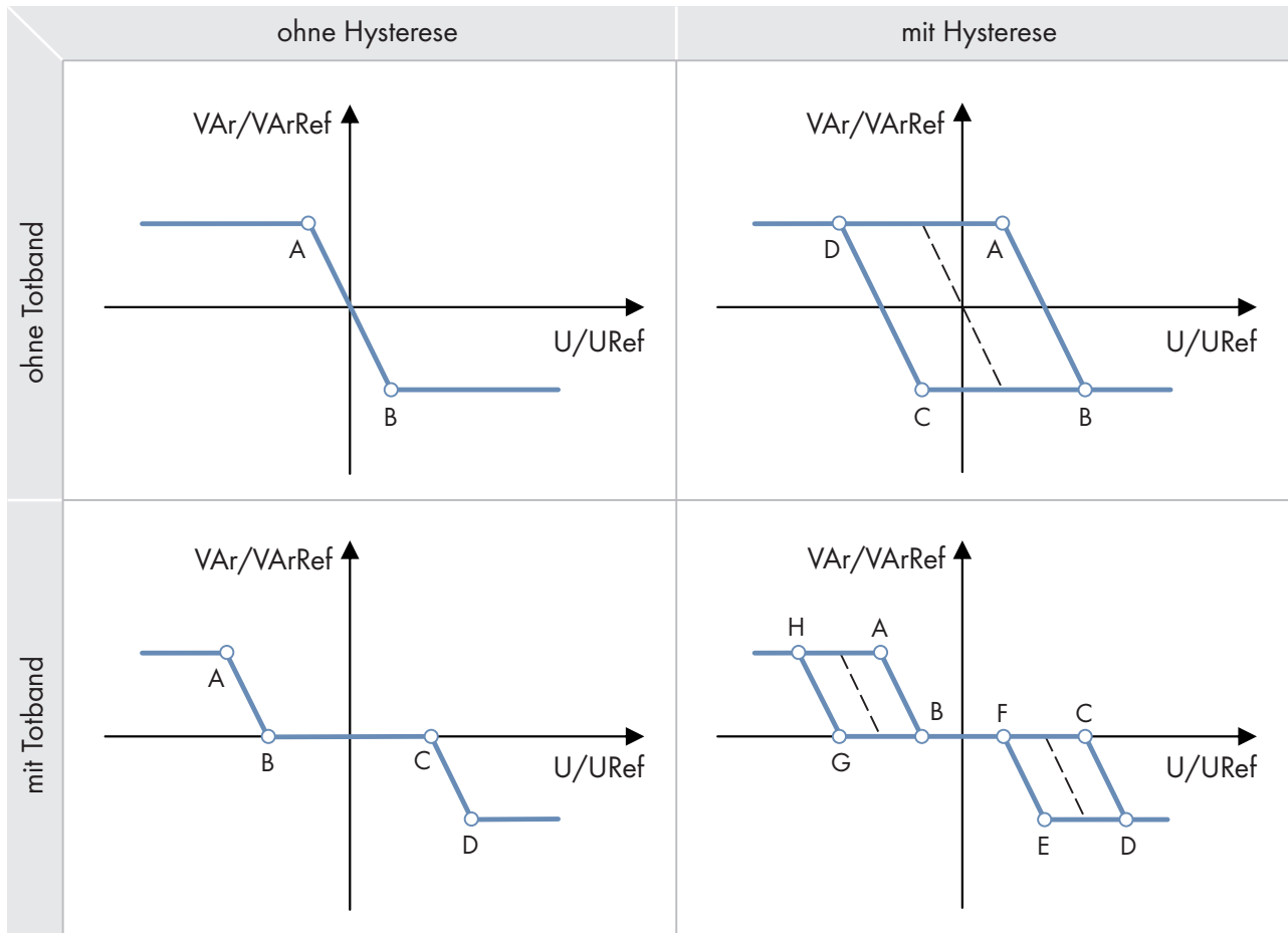
Abbildung 14: Q(U)-Kennlinien (Beispiele)
