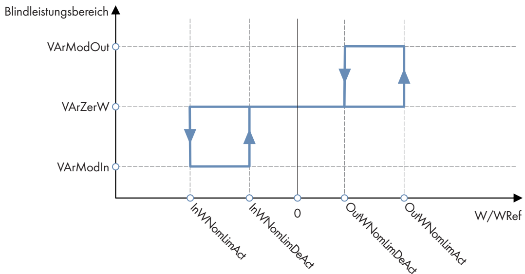
Abbildung 8: Aktivierung / Deaktivierung der Blindleistungsbereiche in Abhängigkeit von der Wirkleistung
