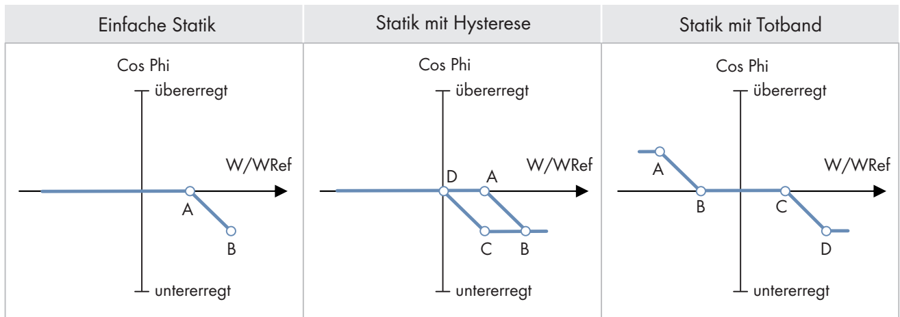
Abbildung 15: Cos-Phi-/Wirkleistungskennlinie Cos Phi(P) (Beispiele)
