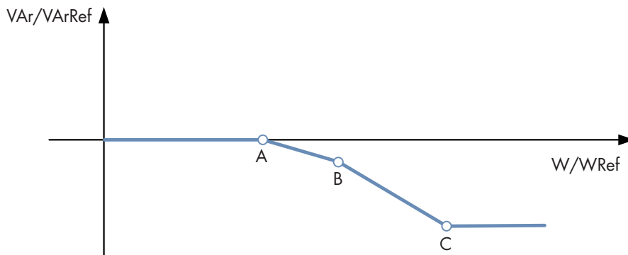
Abbildung 11: Beispiel einer Q(P)-Kennlinie für reine Erzeuger mit 3 Stützpunkten
