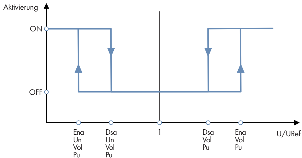
Abbildung 16: Prinzip der spannungsabhängigen Aktivierung
