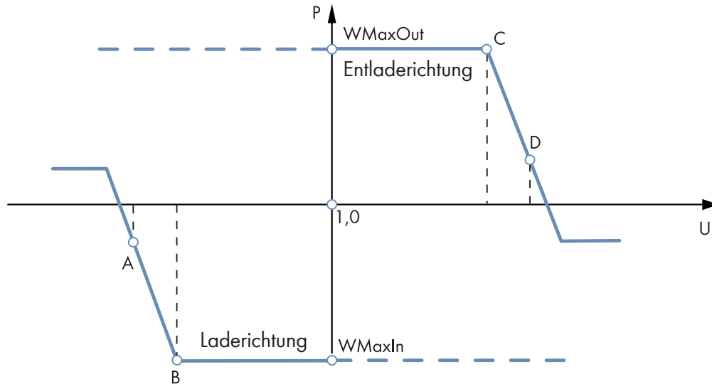
Abbildung 7: Beispiel einer P(U)-Kennlinie mit zwei Stützpunkten, erweitert um Laderichtung
