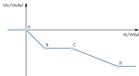
Abbildung 12: Beispiel einer Q(P)-Kennlinie mit 4 Stützpunkten nach IEEE 1547.1 Charakteristik 2-B
