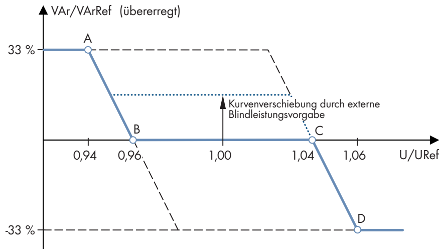
Abbildung 9: Kennlinie für dynamische Sollwertvorgabe mit aktivierter Spannungsbegrenzungsfunktion (Beispiel)
