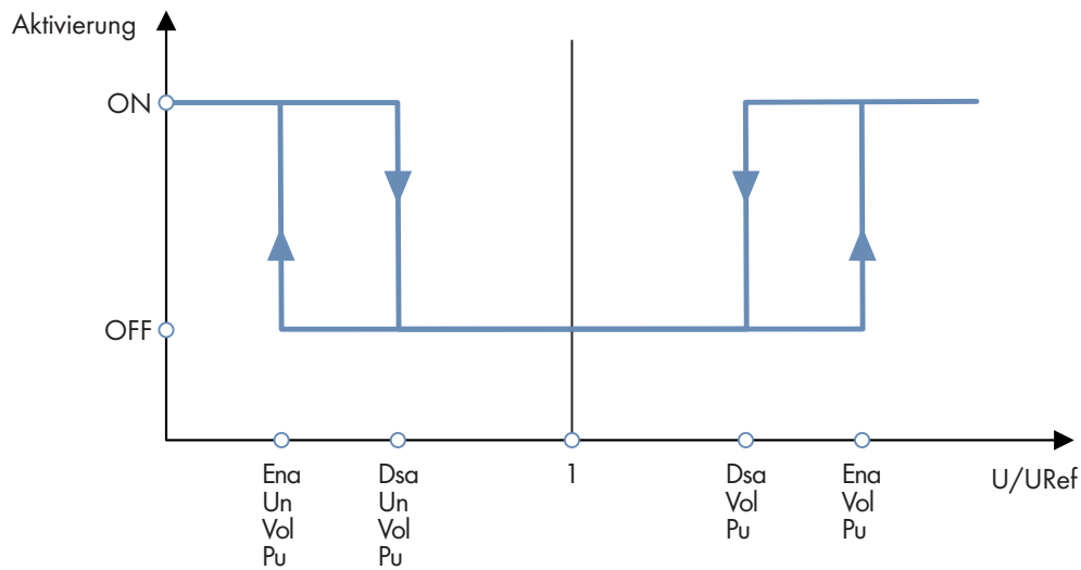
Abbildung 13: Prinzip der spannungsabhängigen Aktivierung
