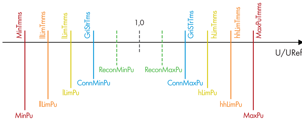
Abbildung 18: Spannungsüberwachung
