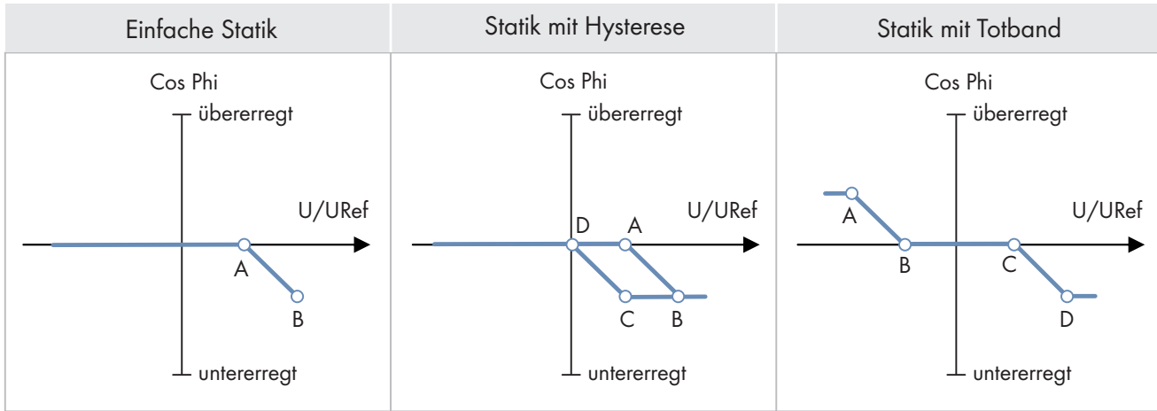
Abbildung 17: Cos-Phi-/Spannungskennlinie Cos Phi(U) (Beispiele)
