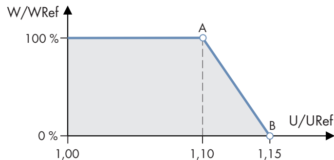
Abbildung 6: Beispiel einer P(U)-Kennlinie mit zwei Stützpunkten
