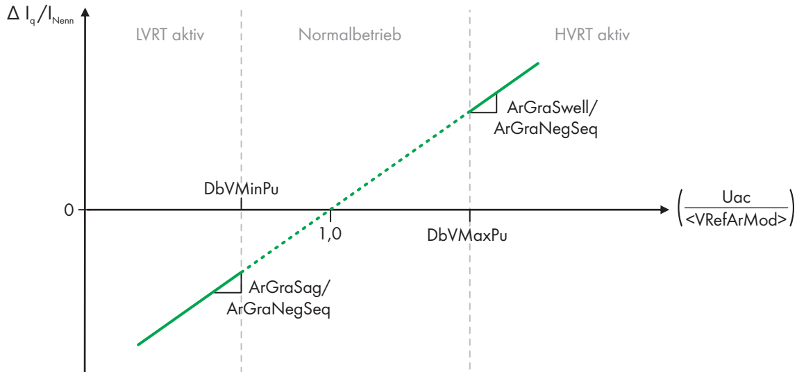
Abbildung 19: Kennlinie der vollständigen dynamischen Netzüberwachung
