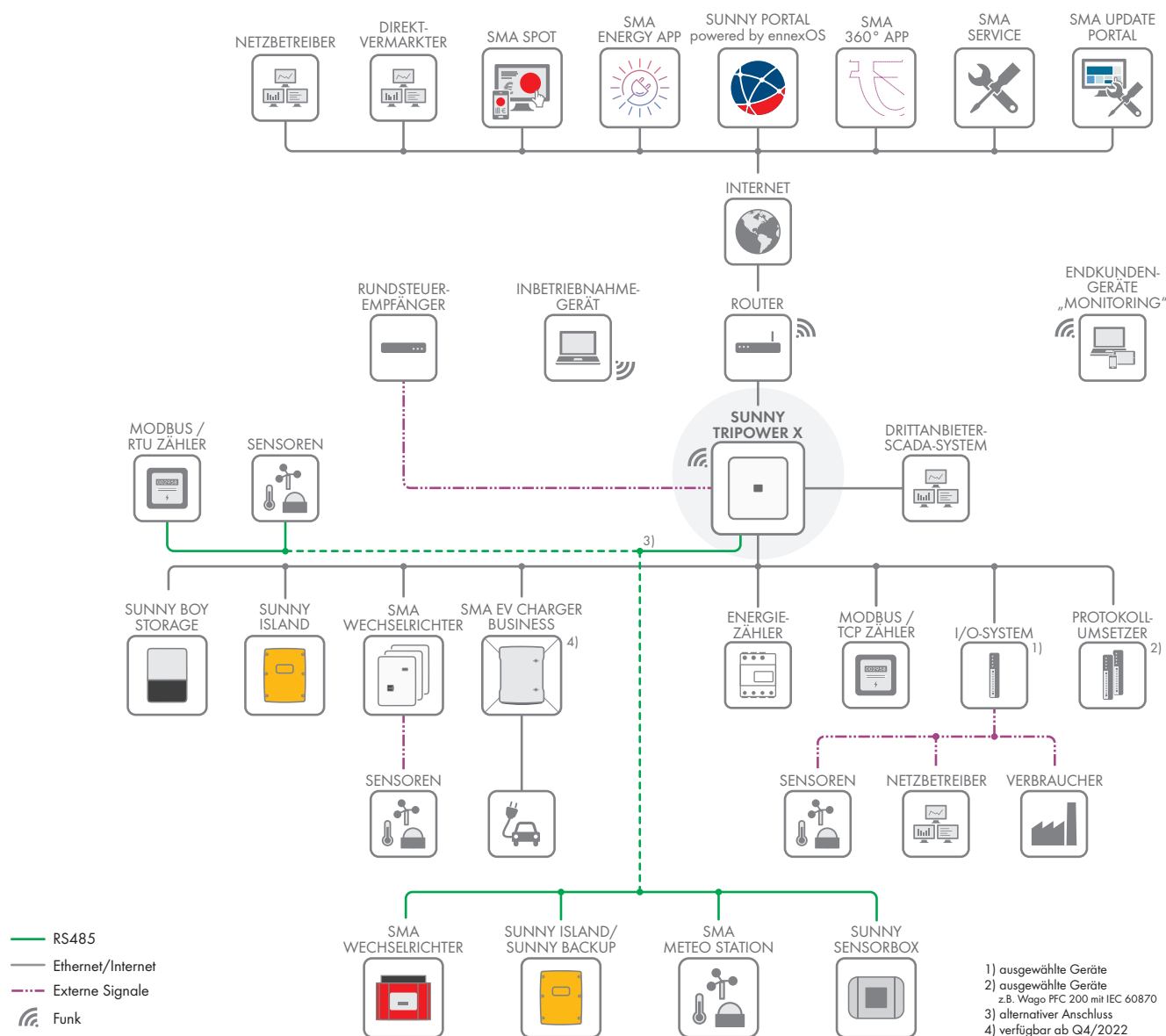
Abbildung 4: Kommunikationsübersicht in Systemen mit Sunny Tripower X als System Manager
